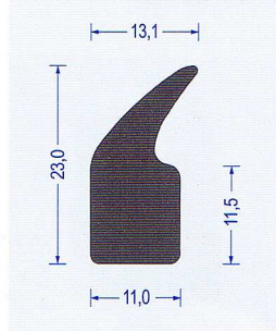
Art.-Nr. 2150003 EPDM schwarz VE : 50 m Bund
