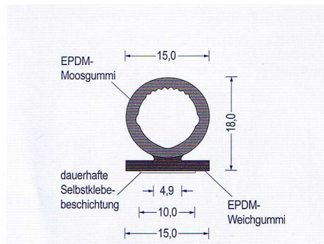
Art.-Nr. 2180002 EPDM schwarz skd* VE : 100 m Bund
