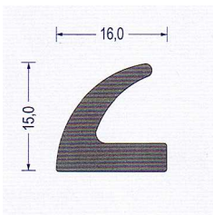
Art.-Nr. 2150016 EPDM - schwarz VE : 25 m Bund
