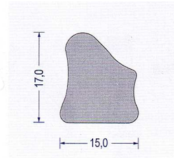
Art.-Nr. 2150013 EPDM - grau VE : 50 m Bund
