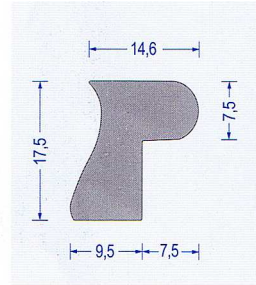
Art.-Nr. 2150007 EPDM grau VE : 50 m Bund
