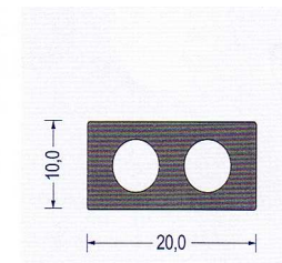
Art.-Nr. 2150018 EPDM schwarz VE : 50 m Bund
