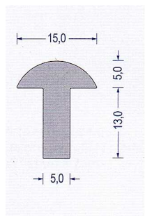
Art.-Nr. 2150021 EPDM grau VE : 50 m Bund
