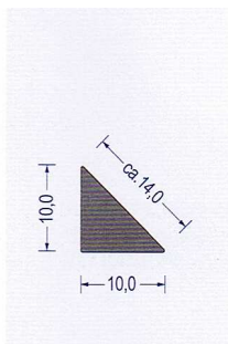
Art.-Nr. 2150022 EPDM grau VE : 50 m Bund
