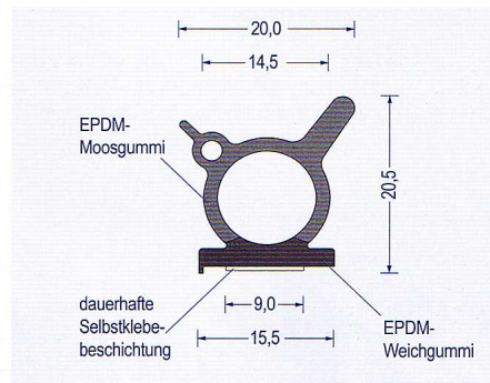
Art.-Nr. 2180003 EPDM schwarz skd* VE : 50 m Bund
