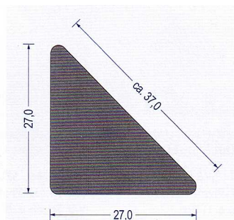
Art.-Nr. 2150024 EPDM schwarz VE : 25 m Bund
