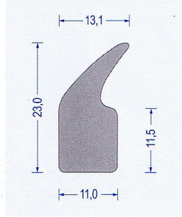
Art.-Nr. 2150002 EPDM grau VE : 50 m Bund
