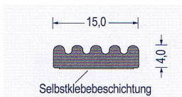
Art.-Nr. 2170006 EPDM schwarz sk* VE : 100 m Spule
