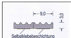
Art.-Nr. 2172001 EPDM(Krone) - grau sk* VE : 140 m Spule Doppelmeter m. Abrißkante
