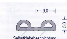
Art.-Nr. 2171001 EPDM(P) - grau sk* VE : 100 m Spule Doppelmeter m. Abrißkante
