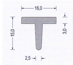
Art.-Nr. 2150012 EPDM - grau VE : 25 m Bund
