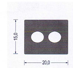
Art.-Nr. 2150019 EPDM schwarz VE : 50 m Bund
