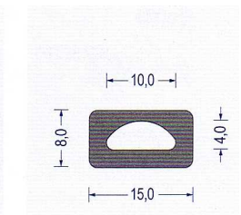
Art.-Nr. 2150020 EPDM schwarz VE : 100 m Bund
