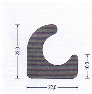
Art.-Nr. 2150025 EPDM schwarz VE : 25 m Bund
