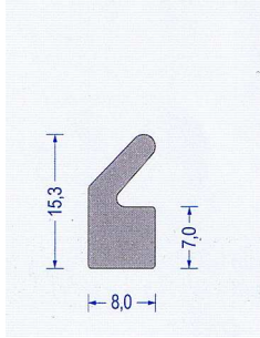
Art.-Nr. 2150001 EPDM grau VE : 50 m Bund
