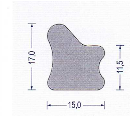
Art.-Nr. 2150015 EPDM grau VE : 50 m Bund
