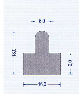
Art.-Nr. 2150004 EPDM grau VE : 50 m Bund
