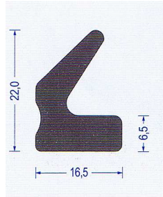
Art.-Nr. 2150006 EPDM schwarz VE : 25 m Bund
