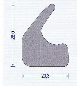
Art.-Nr. 2150008 EPDM grau VE : 25 m Bund
