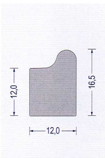
Art.-Nr. 2150023 EPDM grau VE : 50 m Bund
