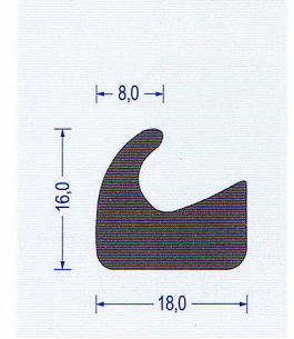
Art.-Nr. 2150005 EPDM schwarz VE : 25 m Bund
