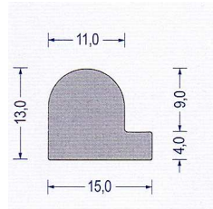
Art.-Nr. 2150011 EPDM - grau VE : 50 m Bund
