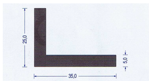
Art.-Nr. 2380005 EPDM 65 schwarz VE : 25 m Bund
