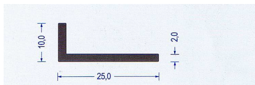
Art.-Nr. 2380001 EPDM 65 schwarz VE : 50 m Bund
