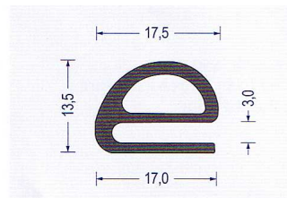
Art.-Nr. 2370006 EPDM 65 schwarz VE : 50 m Bund
