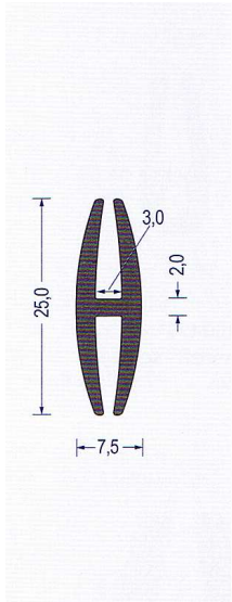
Art.-Nr. 2360001 EPDM 65 schwarz VE : 50 m Bund
