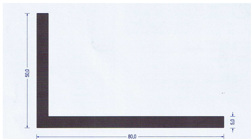
Art.-Nr. 2380008 · EPDM 65 ° Shore A · schwarz · VE Bund à 10 m
