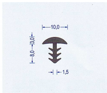
Art.-Nr. 2390002 EPDM 65 schwarz VE : 50 m Bund
