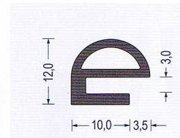
Art.-Nr. 2370004 EPDM 75 schwarz VE : 50 m Bund
