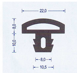
Art.-Nr. 2390003 EPDM 65 schwarz VE : 50 m Bund
