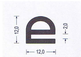
Art.-Nr. 2370003 EPDM 65 schwarz VE : 50 m Bund
