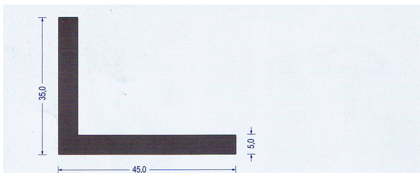
Art.-Nr. 2380006 · EPDM 65 ° Shore A · schwarz · VE Bund à 15 m
