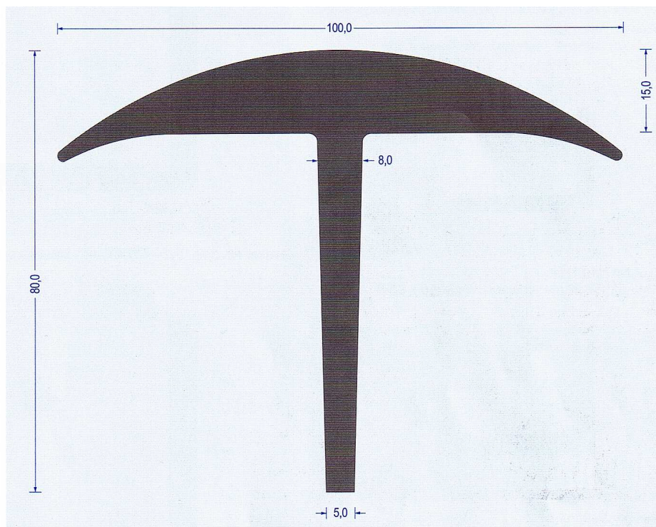
Art.-Nr. 2390005 EPDM 65 schwarz VE : 18,1 m Bund
