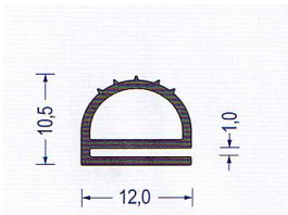
Art.-Nr. 2370001 EPDM 65 schwarz VE : 50 m Bund
