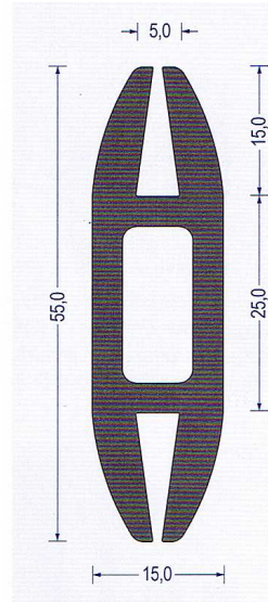
Art.-Nr. 2360004 EPDM 65 schwarz VE : 26 m Bund
