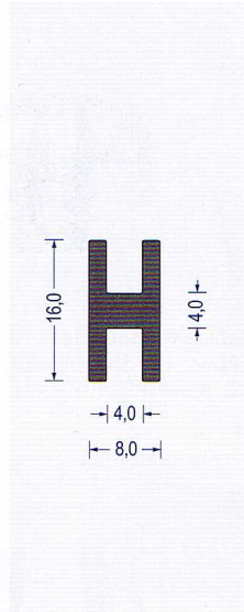
Art.-Nr. 2360003 EPDM 65 schwarz VE : 50 m Bund
