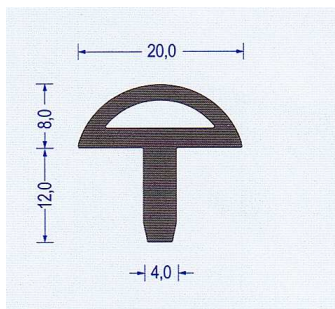
Art.-Nr. 2390001 EPDM 65 schwarz VE : 50 m Bund
