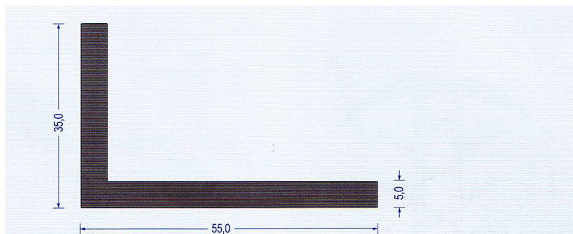
Art.-Nr. 2380007 · EPDM 65 ° Shore A · schwarz · VE Bund à 15 m
