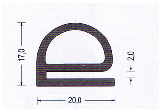
Art.-Nr. 2370005 EPDM 65 schwarz VE : 50 m Bund
