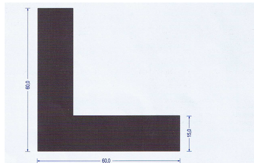
Art.-Nr. 2380009 · EPDM 65 ° Shore A · schwarz · VE Bund à 4 m
