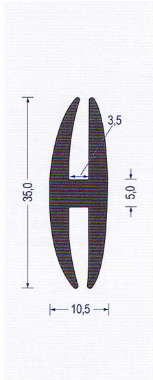
Art.-Nr. 2360002 EPDM 65 schwarz VE : 50 m Bund
