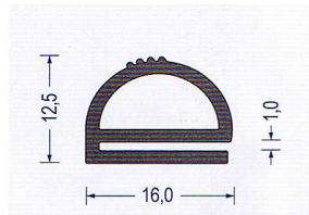
Art.-Nr. 2370002 EPDM 65 schwarz VE : 50 m Bund
