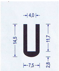
Art.-Nr. 2300060 EPDM 60 schwarz VE : 100 m Bund
