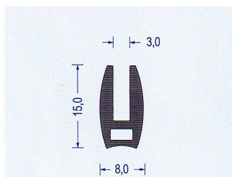
Art.-Nr. 2310003 EPDM 65 schwarz VE : 50 m Bund
