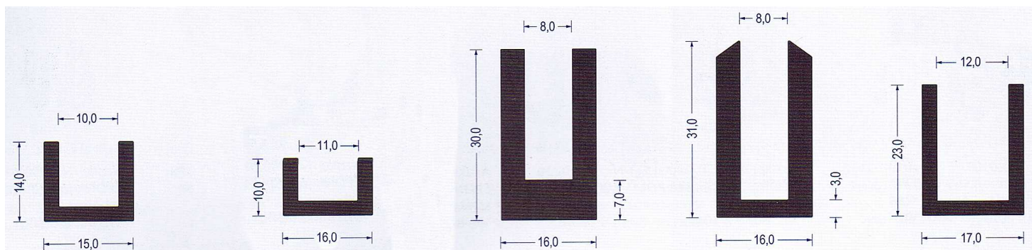
Art.-Nr. 2300029 EPDM 65 schwarz VE : 50 m Bund
