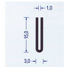
Art.-Nr. 2300058 EPDM 65 schwarz VE : 100 m Bund
