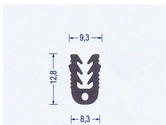
Art.-Nr. 2310002 EPDM 65 schwarz VE : 50 m Bund
