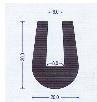
Art.-Nr. 2310010 EPDM 65 schwarz VE : 25 m Bund
