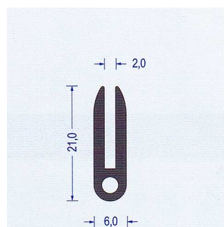
Art.-Nr. 2310005 EPDM 45 schwarz VE : 100 m Bund
