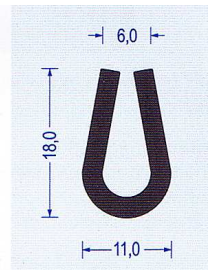
Art.-Nr. 2300064 EPDM 65 schwarz VE : 100 m Bund
