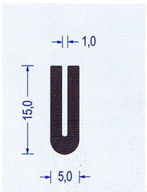
Art.-Nr. 2300059 EPDM 55 schwarz VE : 100 m Bund
