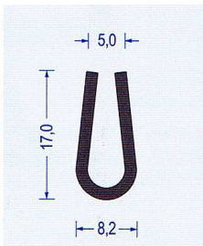
Art.-Nr. 2300061 EPDM 65 schwarz VE : 100 m Bund
