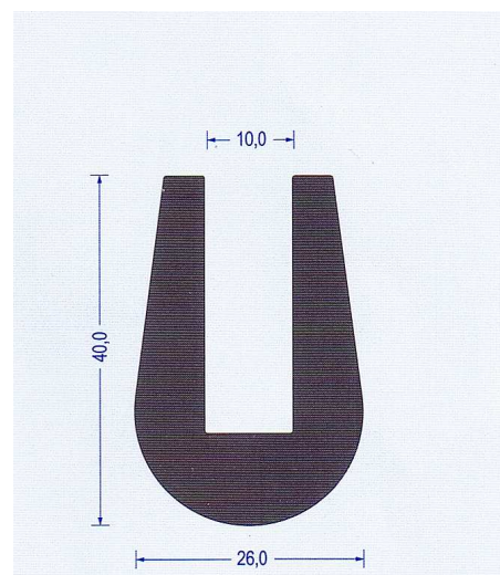
Art.-Nr. 2310012 EPDM 65 schwarz VE : 25 m Bund
