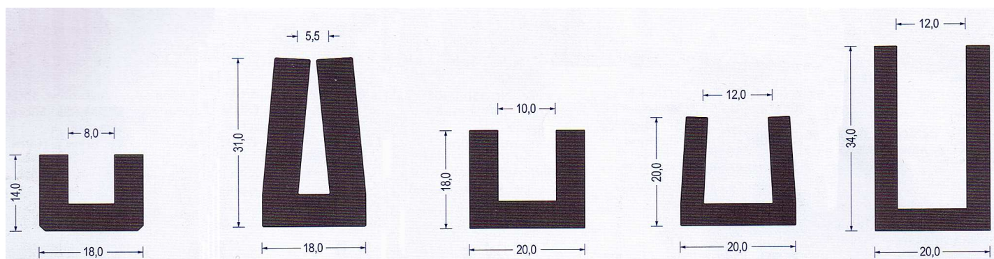
Art.-Nr. 2300034 SBR 60 schwarz VE : 35 m Bund
