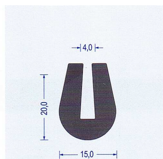
Art.-Nr. 2310006 EPDM 65 schwarz VE : 50 m Bund
