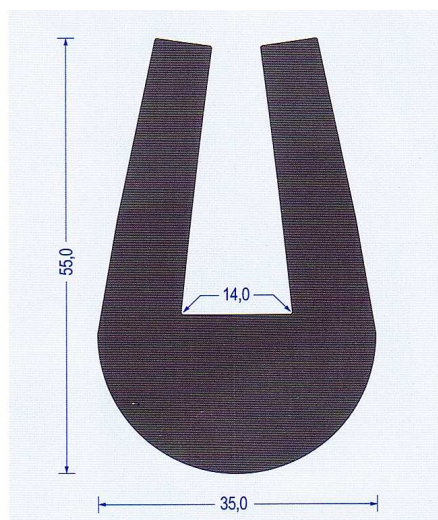
Art.-Nr. 2310013 EPDM 65 schwarz VE : 25 m Bund
