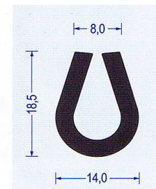
Art.-Nr. 2300066 EPDM 70 schwarz VE : 50 m Bund
