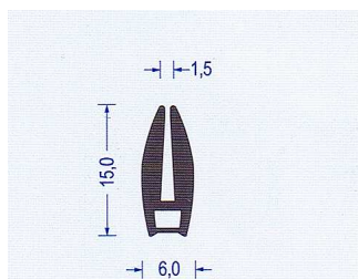
Art.-Nr. 2310001 EPDM 65 schwarz VE : 100 m Bund
