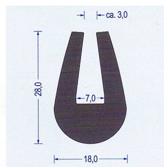
Art.-Nr. 2310008 EPDM 70 schwarz VE : 25 m Bund
