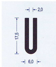
Art.-Nr. 2300062 EPDM 65 schwarz VE : 50 m Bund
