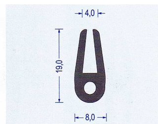
Art.-Nr. 2310004 EPDM 65 schwarz VE : 50 m Bund
