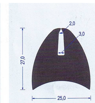
Art.-Nr. 2310011 EPDM 55 schwarz VE : 25 m Bund
