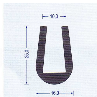
Art.-Nr. 2310007 EPDM 45 schwarz VE : 50 m Bund
