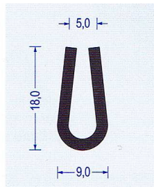
Art.-Nr. 2300063 EPDM 65 schwarz VE : 100 m Bund
