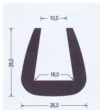
Art.-Nr. 2310009 EPDM 85 schwarz VE : 25 m Bund
