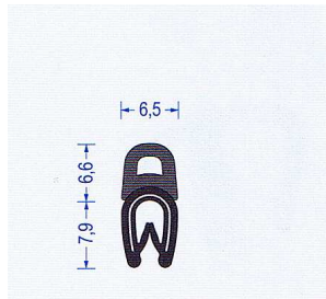
Art.-Nr. 2810013 schwarz Klemmbereich 1-2 mm VE: 100 m Bund Br* a40/b40/c10/d10
