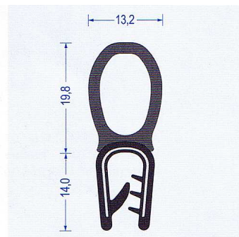
Art.-Nr. 2810023 schwarz Klemmbereich 2-4 mm VE: 50 m Bund Br* a80/b100/c20/d20
