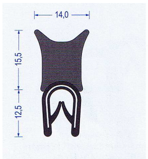
Art.-Nr. 2810017 schwarz Klemmbereich 1-4 mm VE: 50 m Bund Br* a50/b150/c50/d50
