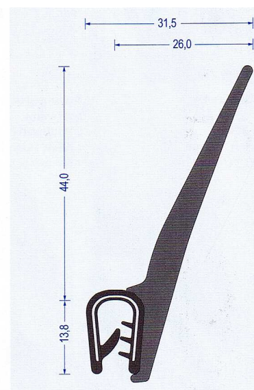
Art.-Nr. 2810029 schwarz Klemmbereich 4-6 mm VE: 25 m Bund Br* a80/b-c120/d120
