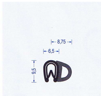
Art.-Nr. 2810018 schwarz Klemmbereich 1-2 mm VE: 100 m Bund Br* a20/b15/c30/d50
