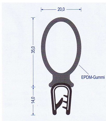
Art.-Nr. 2810026 schwarz Klemmbereich 2-4 mm VE: 25 m Bund Br* a100/b160/c40/d40
