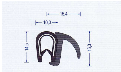
Art.-Nr. 2810001 · schwarz Klemmber.1-4 mm · VE: 50 m Bund Br* a40/b40/c150/d150
