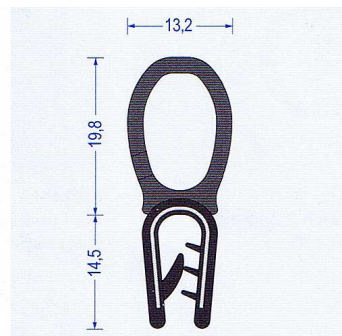
Art.-Nr. 2810022 schwarz Klemmbereich 1-2,5 mm VE: 50 m Bund Br* a80/b100/c20/d20
