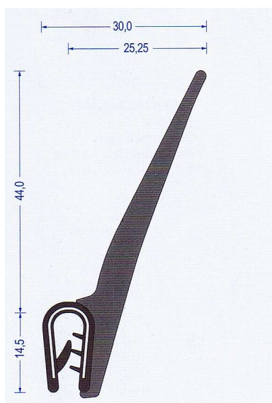
Art.-Nr. 2810027 schwarz Klemmbereich 1-2 mm VE: 25 m Bund Br* a80/b-c120/d120
