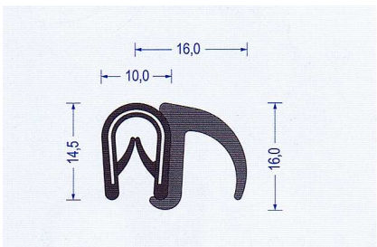
Art.-Nr. 2810004 · schwarz Klemmber.1-4 mm · VE: 50 m Bund Br* a40/b40/c150/d150
