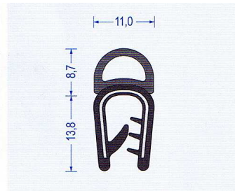
Art.-Nr. 2810015 schwarz Klemmbereich 4-6 mm VE: 50 m Bund Br* a90/b100/c40/d40
