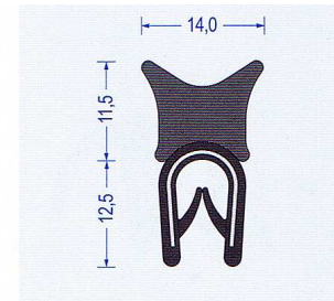
Art.-Nr. 2810016 schwarz Klemmbereich 1-4 mm VE: 50 m Bund Br* a50/b150/c50/d50
