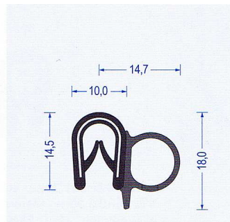
Art.-Nr. 2810019 schwarz Klemmbereich 1-4 mm VE: 50 m Bund Br* a50/b40/c60/d120
