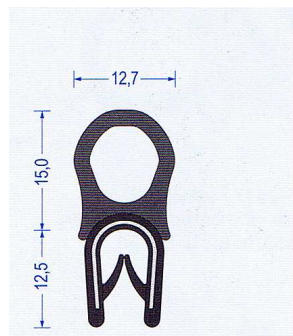
Art.-Nr. 2810021 schwarz Klemmbereich 1-4 mm VE: 50 m Bund Br* a60/b80/c20/d20
