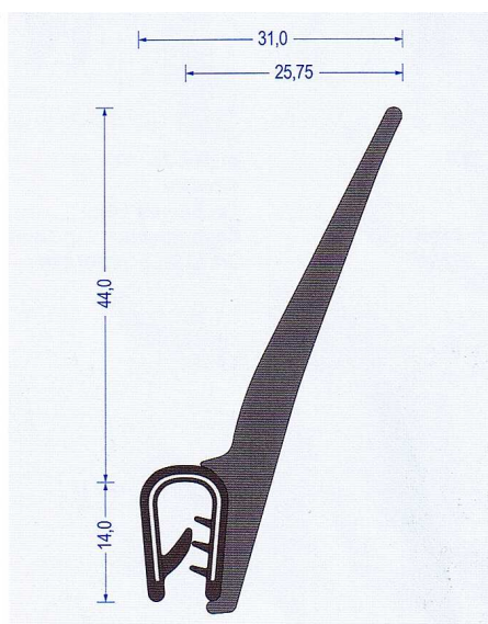
Art.-Nr. 2810028 schwarz Klemmbereich 2,5-4 mm VE: 25 m Bund Br* a80/b-c120/d120
