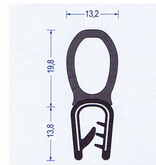
Art.-Nr. 2810024 schwarz Klemmbereich 4-6 mm VE: 50 m Bund Br* a80/b100/c20/d20
