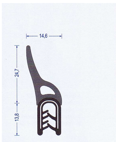
Art.-Nr. 2810025 schwarz Klemmbereich 1,5-3,5 mm VE: 50 m Bund Br* a80/b150/c30/d30
