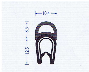
Art.-Nr. 2810014 schwarz Klemmbereich 1-4 mm VE: 50 m Bund Br* a70/b80/c15/d15
