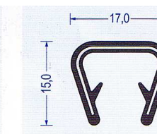
Art.-Nr. 2800026 schwarz Klemmber. 9 - 12 mm VE : 100 m Bund Br* a50/b20/c20/d20
