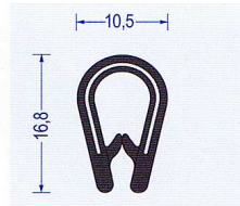
Art.-Nr. 2800015 schwarz Klemmber. 2 - 4 mm VE : 100 m Bund Br* a40/b30/c20/d20
