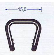
Art.-Nr. 2800025 schwarz Klemmber. 8 - 10 mm VE : 100 m Bund Br* a40/b40/c40/d40
