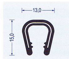
Art.-Nr. 2800023 schwarz Klemmber. 6 - 8 mm VE : 100 m Bund Br* a40/b40/c40/d40
