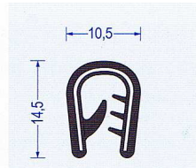
Art.-Nr. 2800016 schwarz Klemmber. 2 - 5 mm VE : 100 m Bund Br* a40/b40/c20/d20
