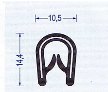
Art.-Nr. 2800014 schwarz Klemmber. 1 - 4 mm VE : 100 m Bund Br* a30/b20/c20/d20
