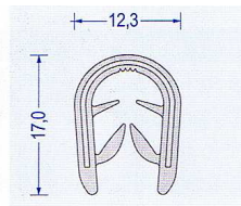
Art.-Nr. 2800020 hellgrau Klemmber. 4 - 6 mm VE : 100 m Bund Br* a45/b30/c15/d15
