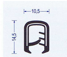
Art.-Nr. 2800017 schwarz Klemmber. 2 - 5 mm VE : 100 m Bund Br* a40/b40/c20/d20
