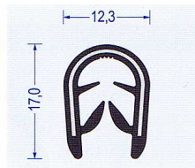
Art.-Nr. 2800021 schwarz Klemmber. 4 - 6 mm VE : 100 m Bund Br* a45/b30/c15/d15
